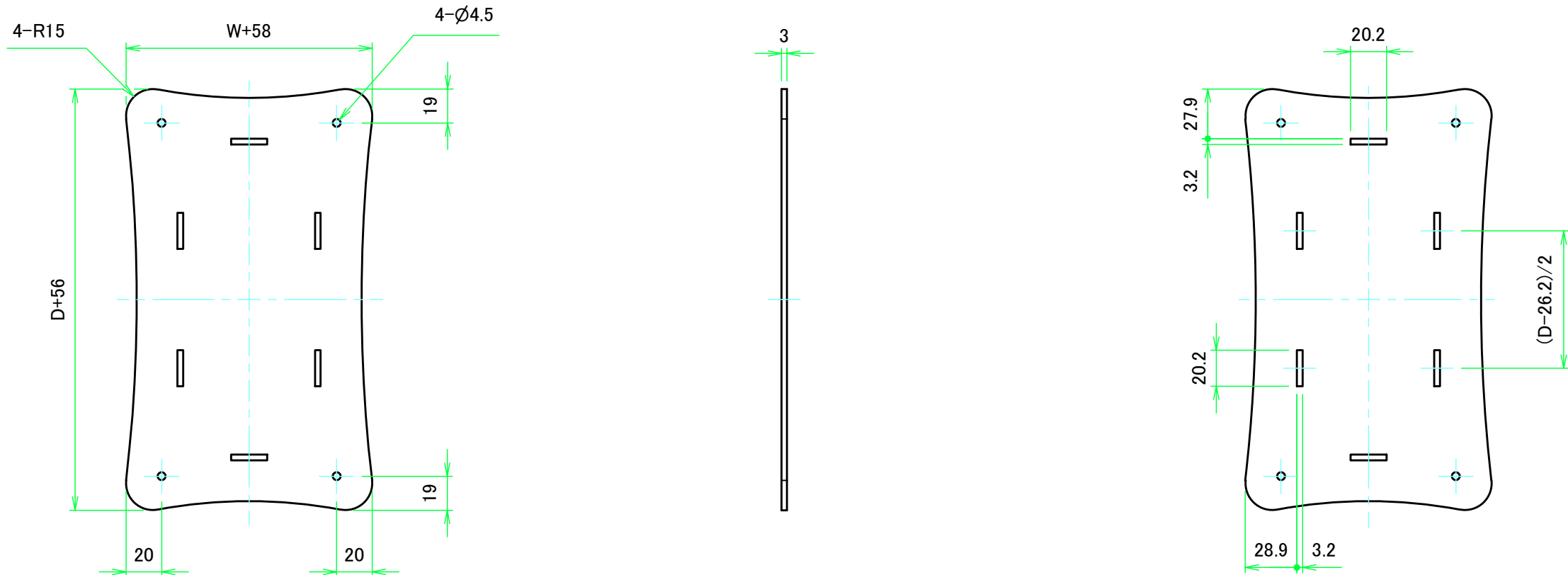
上カバー表面 / Top cover Frontside
