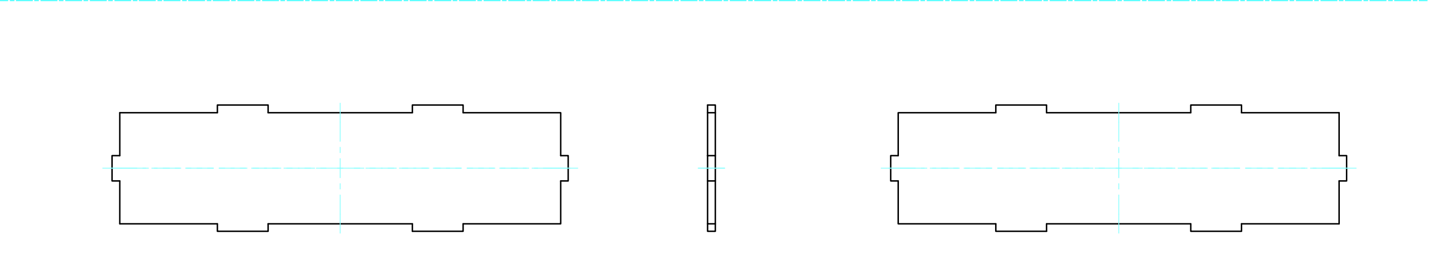
Dパネル1表面 / D panel 1 Frontside
